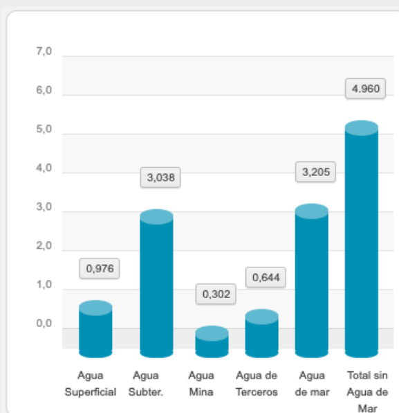
Extracción de agua Región de Antofagasta Gran Minería año 2017 (m3/s)
