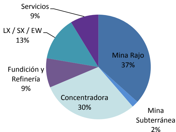
Consumo energético por procesos Total 169.918 TJ
