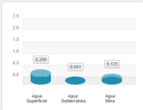
Extracción de agua Región Metropolitana Gran Minería 2014, por cuenca (m3/s)
