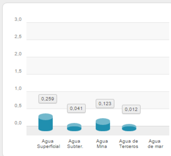
Extracción de agua Región Metropolitana Gran Minería año 2014 (m3/s)
