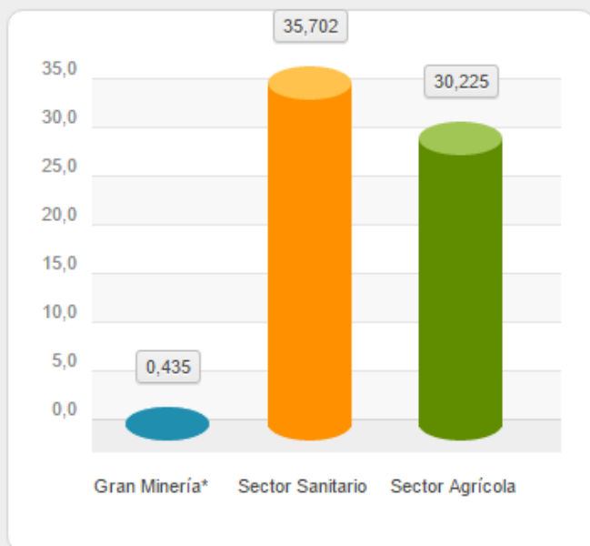
Extracción de agua Región Metropolitana por sector año 2014 (m3/s)
