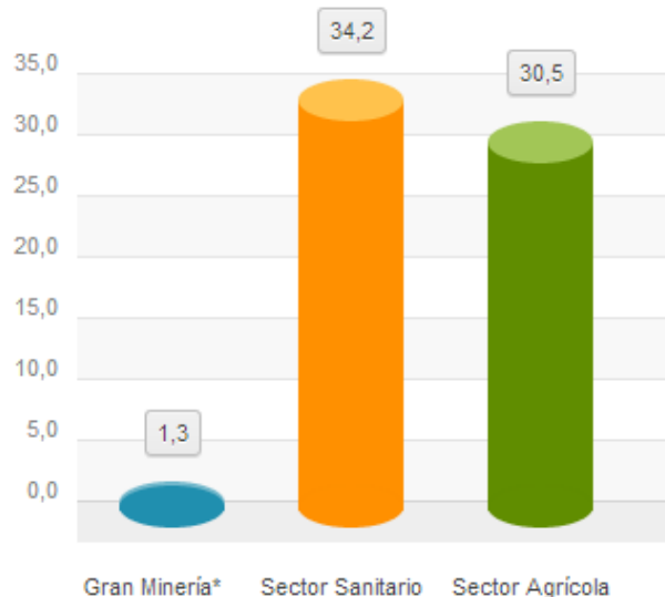
Extracción de agua Región Metropolitana por sector año 2013 (m3/s)
