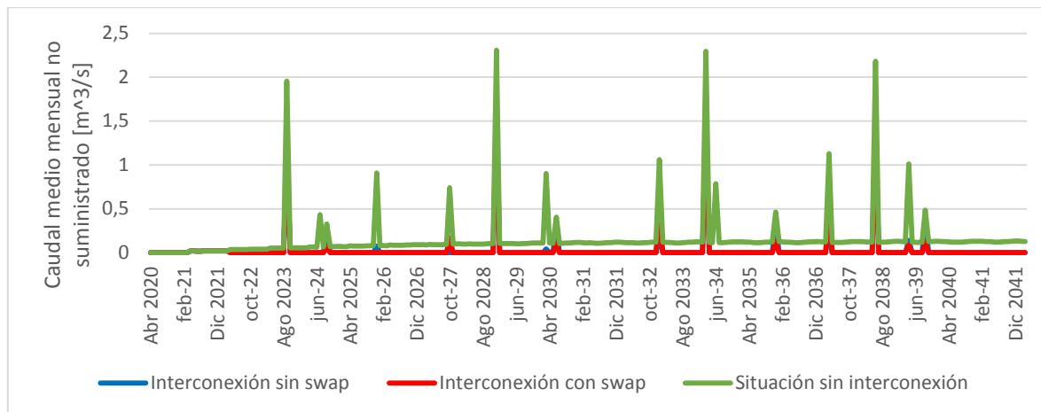
Figura 6.7. Caudal medio mensual no suministrado en el caso con un 20% del aumento de la demanda [ m^3/s ].
